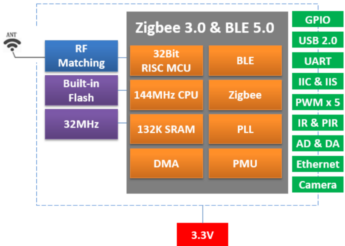
Fig.1.1 XT-ZB6 Module Structure
