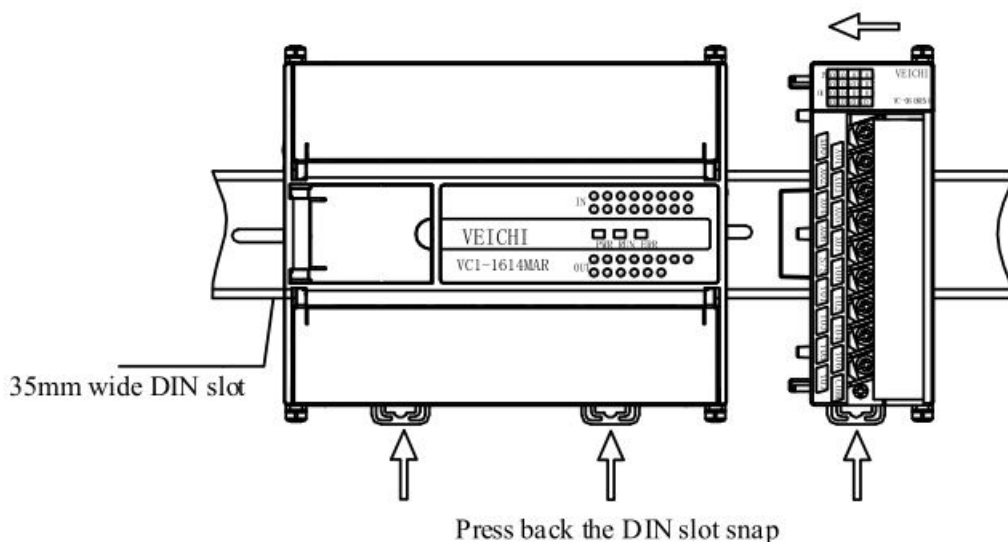
Fig. 6-2 Fixing with DIN slot
