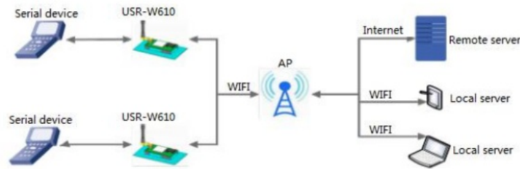
Figure 6 STA mode
