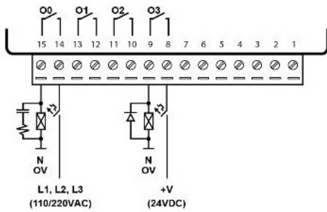
JZ20-R10/JZ20-J-R10
