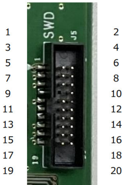
Fig. 4.10. Debugger Connector (J5)
