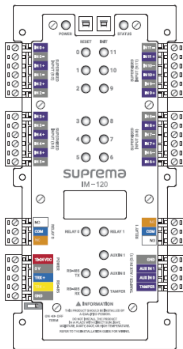
Input Module (IM-120)
