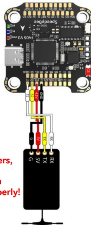
F405 V3 Front Side
