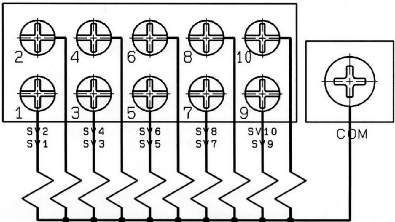
Fig. 3 Valve output wiring
