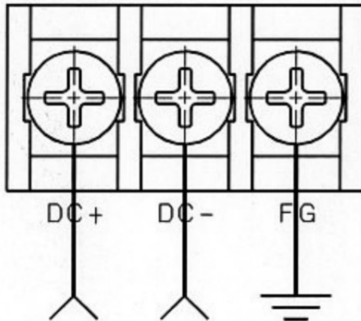
Fig. 2. Wiring diagram
