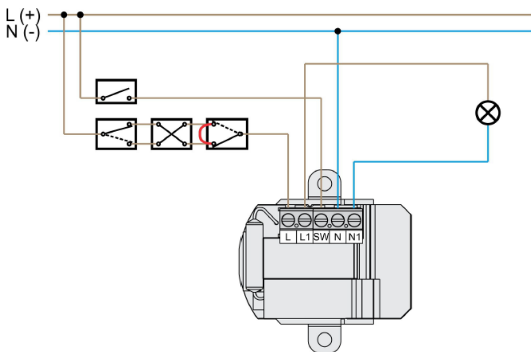
Figure 5: LBT-1.DO1 module
