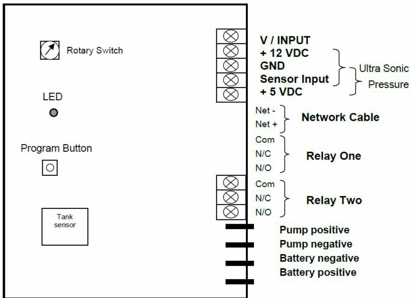
HB-200 Input/Output Unit
