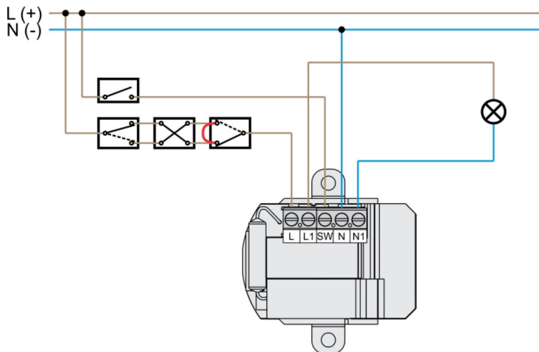
Figure 5: LBT-1.DO1 module
