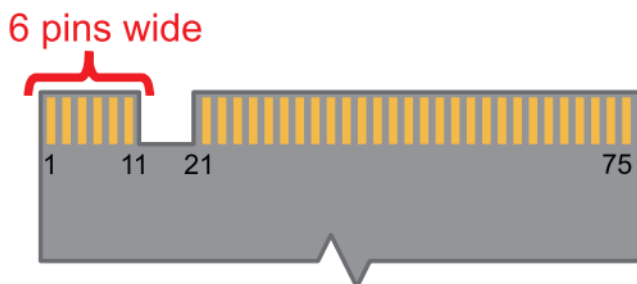
"B key" edge connector
