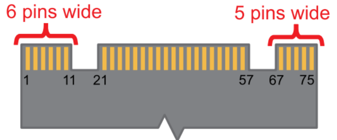
"B & M key" edge connector
