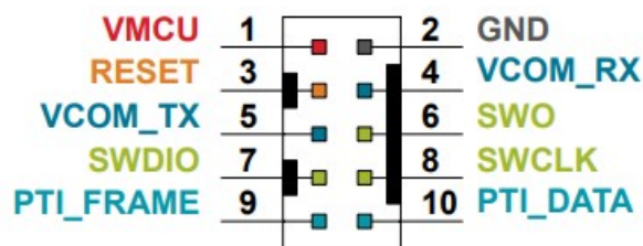
Figure 3.6. Mini Simplicity Connector
