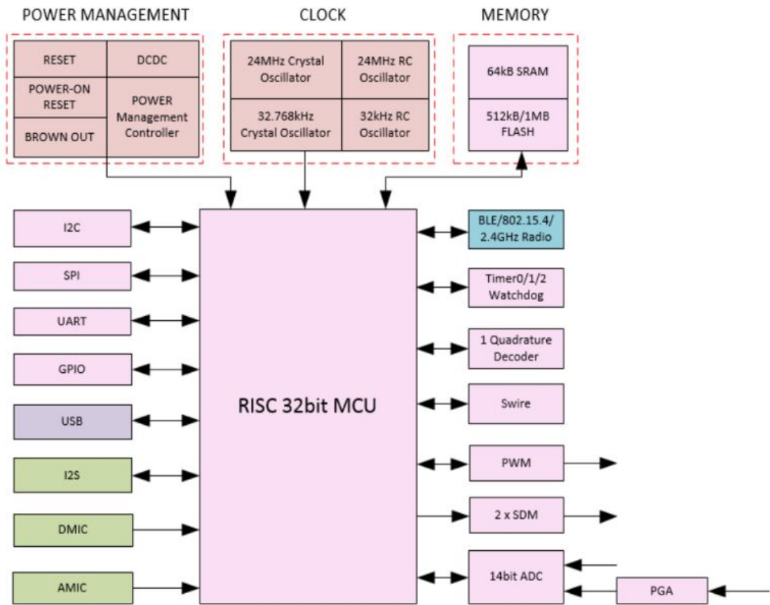
TLS825xSoCdiagram
