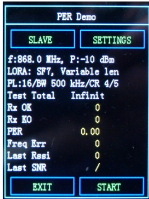
Figure 6: PER Demo Slave Display
