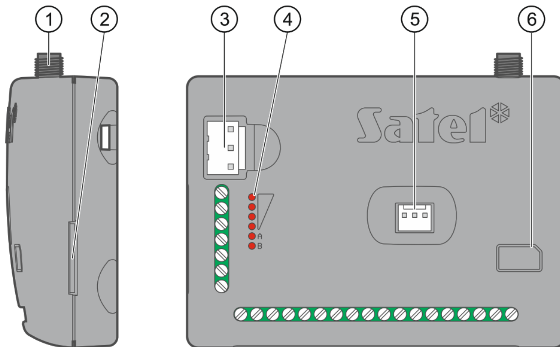
Fig. 1. GPRS-A module.
