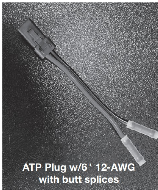
Solar Input
