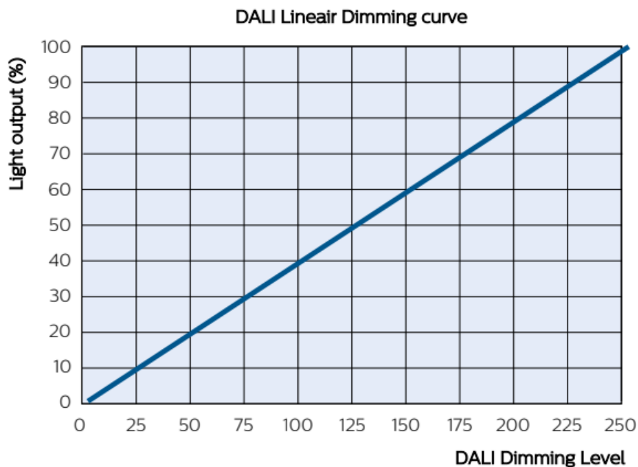
DALI Linear dimming curve
