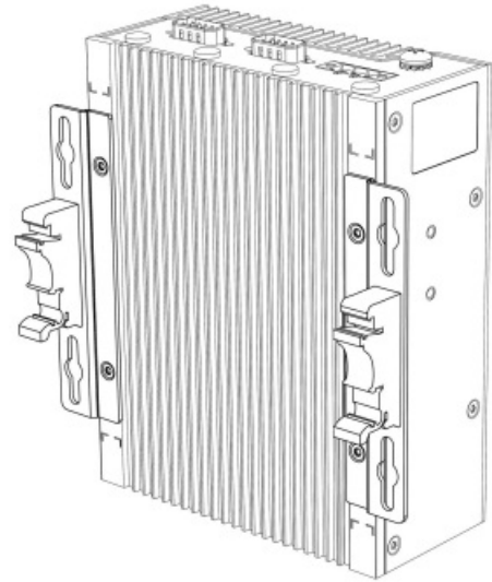
DIN Rail Back Mounting
