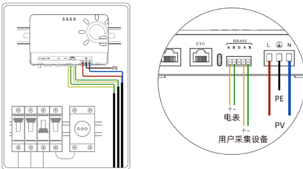
Fig. 3 wiring diagram
