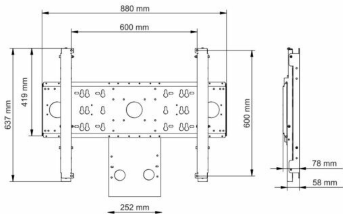
AFL55-800BL1
