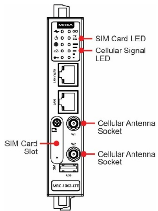
MRC-1002-LTE
