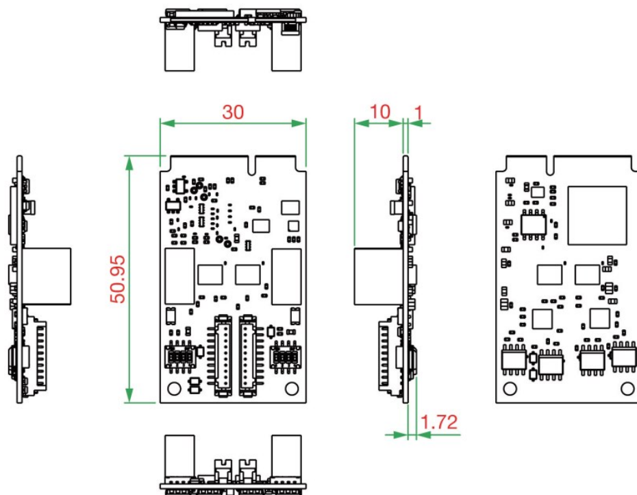
CP-104N-T
