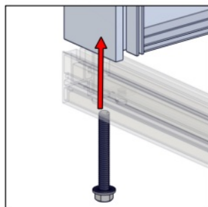
MFY-BOLT-375-16-2.5
