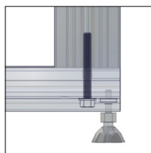
MFY-BOLT-375-16-2.5
