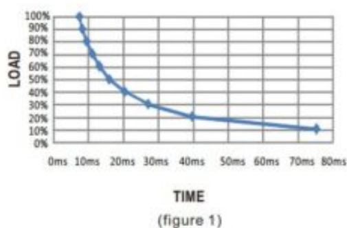
DDR-240C-24
