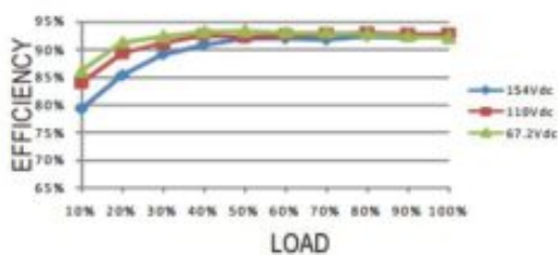
DDR-240D-24
