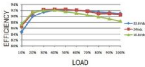
DDR-240B-24
