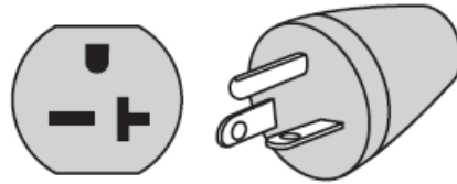
220 NEMA 6-20P PLUG (N.A.)
