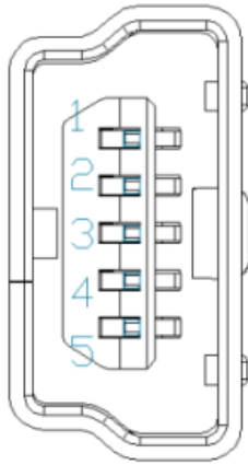
Figure 10: Mini USB Connector
