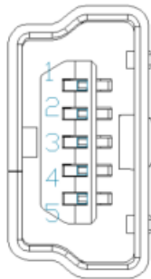
Figure 10: Mini USB Connector
