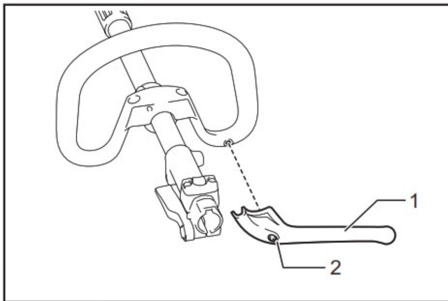
► 1. Barrier 2. Screw
