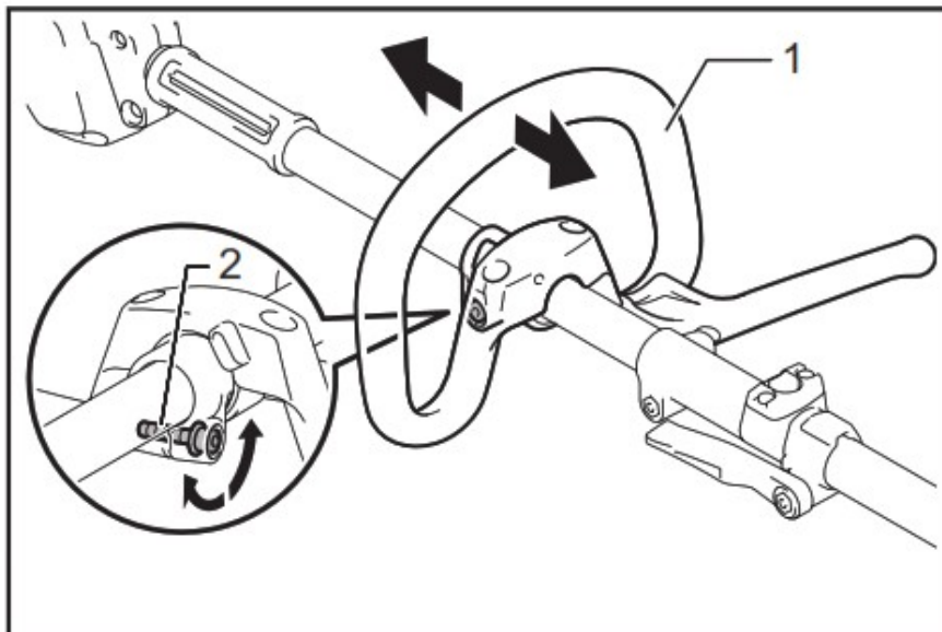
► 1. Handle 2. Hex socket head bolt
