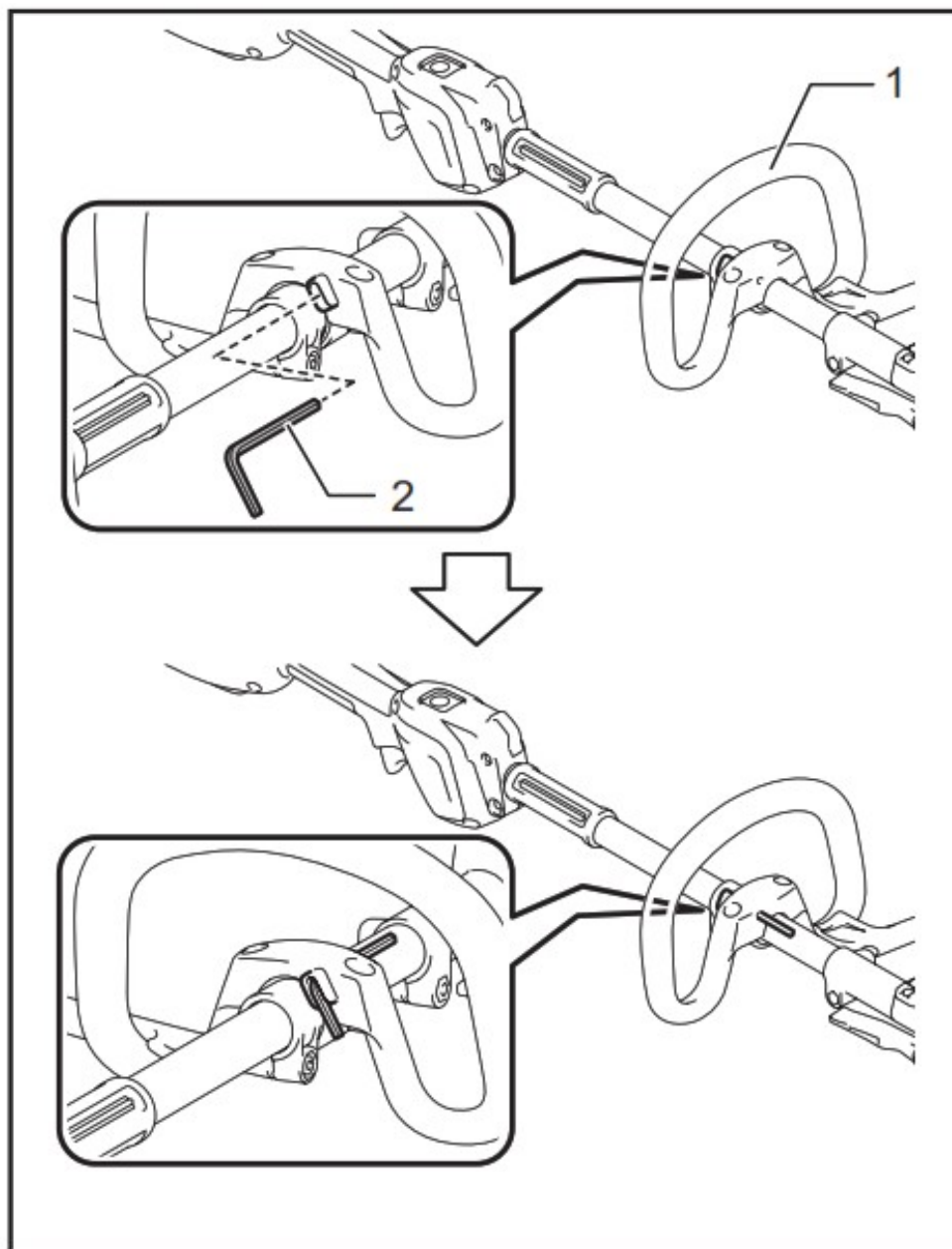
► 1. Handle 2. Hex wrench
