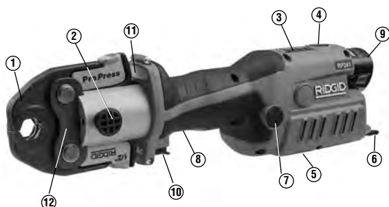
Figura 2 – Selladora RP 241 y mordaza de la serie Compact
