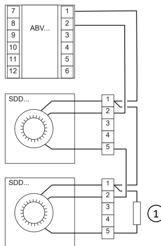
Figur 2 Inkoppling SDD-S65-OE till ABV... Note: –RAC-modellerna får ej kopplas i serie eller till en kontrollenhet.
