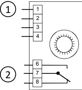
Bild 3 Verdrahtung
