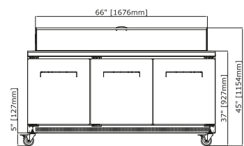
EDST72-18-B Front
