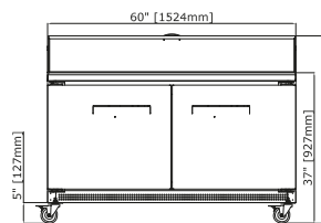
EDST60-16-B Front
