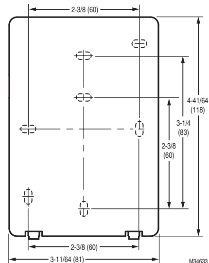
Fig. 2. Orificios de montaje y lengüetas de enganche de la subbase.
