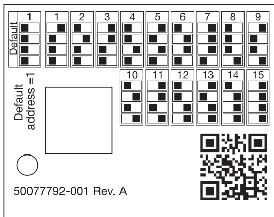
Fig. 7. Etiqueta de configuración de la dirección de bus.
