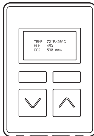
Fig. 11. Pantalla 3 de inicio de visualización LCD del módulo de pared TR42.
