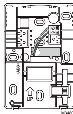
Fig. 6. Conexiones de los terminales.
