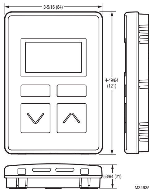
Fig. 4. Dimensiones del módulo de pared con pantalla LCD en pulgadas (mm).
