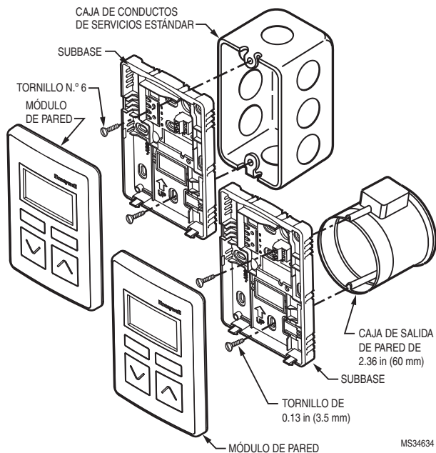
Fig. 3. Instalación en una caja de conductos de servicios estándar o en una caja de salida de pared de 2.36 in (60 mm).
