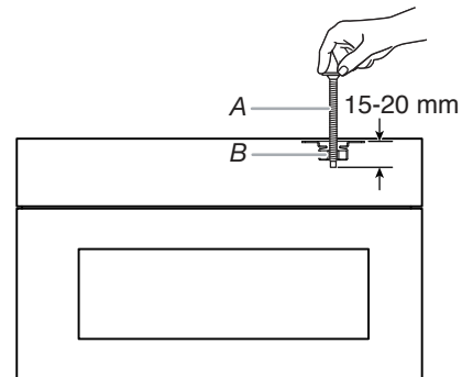
A. Vis B. Écrou de montage
