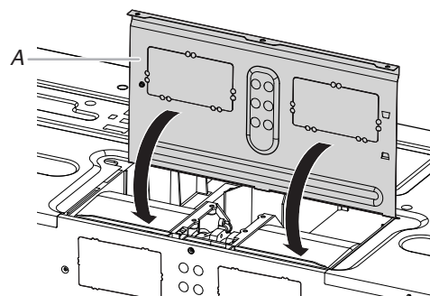
A. Plaque de support du clapet
