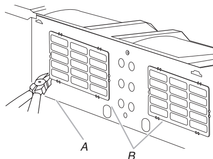
A. Pince coupante diagonale B. Couvercles de fermeture rectangulaire du clapet antiretour
