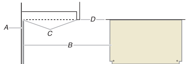
A. Mur arrière B. Plaque de carton C. Le haut de la plaque de carton doit s'aligner avec le bord avant de l'armoire D. Bord avant de l'armoire supérieure
