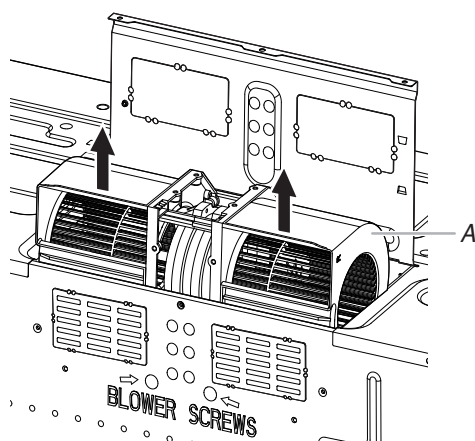
A. Moteur de ventilateur
