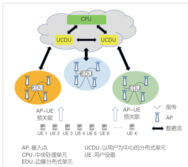
▲图1 新型无蜂窝接入网架构模型图
