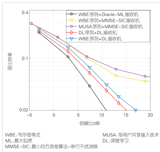
▲图5 智能免授权码本接收机与传统收发算法性能对比
