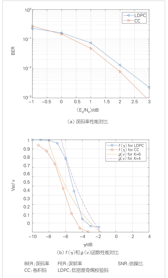
▲图10 卷积码和LDPC性能
