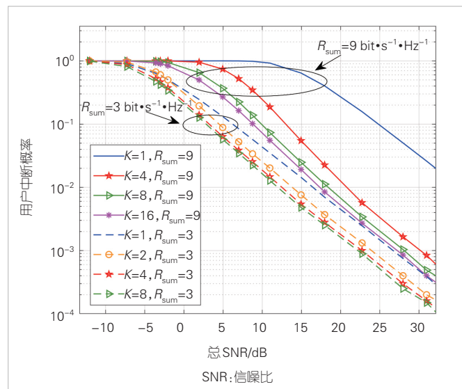
▲图 5 Rayleigh 衰落多址信道的用户平均中断概率 [15]
