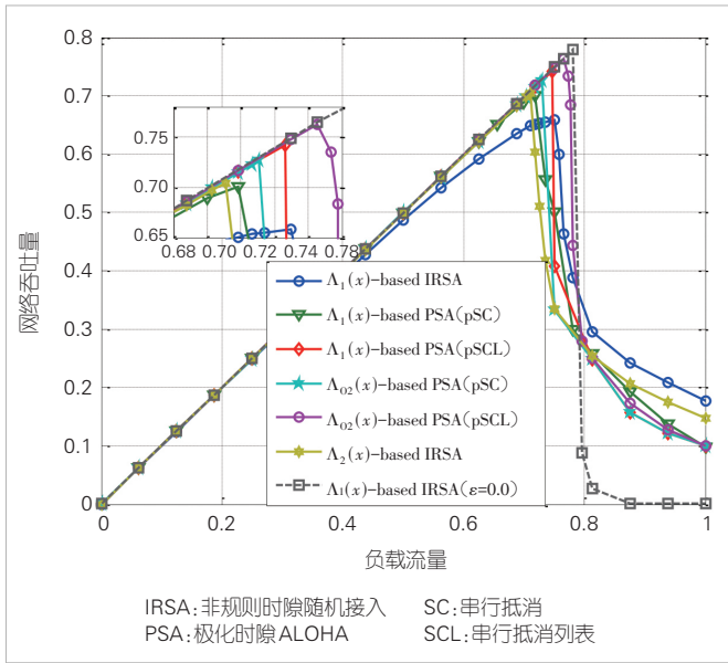
▲图7 PSA随机接入方案经时隙擦除信道传输的系统吞吐量随输入负载变化的性能对比图
