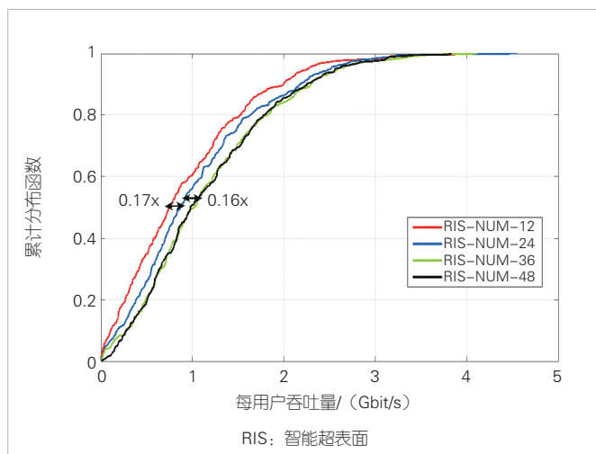
▲图7 不同RIS数目下Het-LDN的每用户吞吐量的累计分布函数(CDF)曲线
