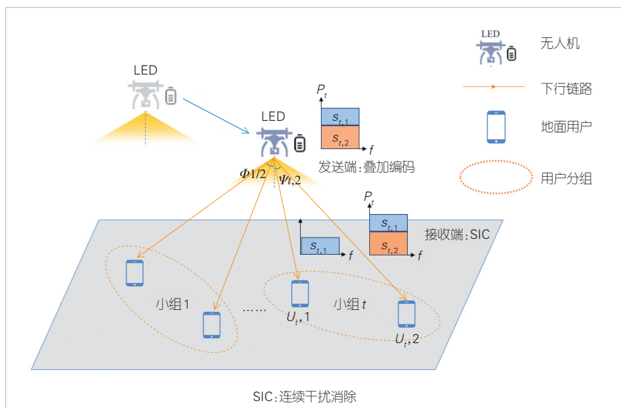
▲图4 无人机辅助可见光通信-非正交多址(VLC-NOMA)系统
