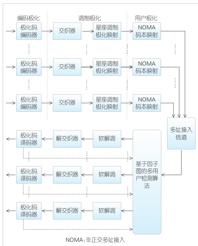
▲图3 极化编码NOMA系统结构
