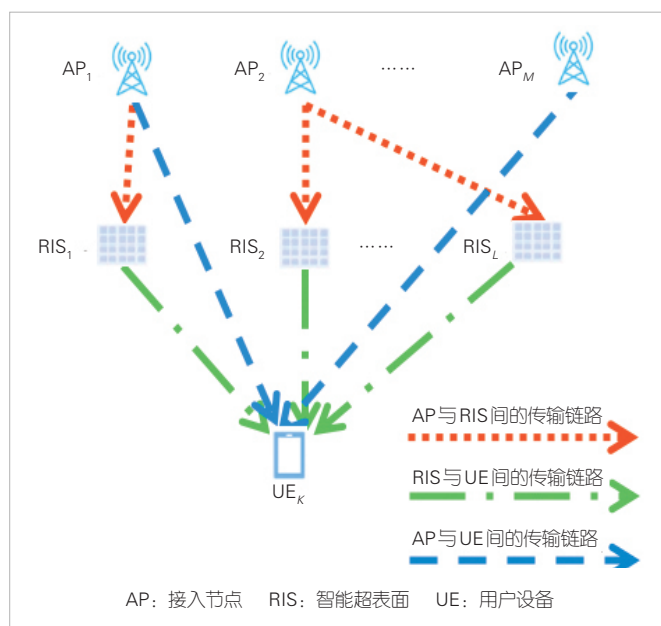
▲图3 Het-LDN传输模型示意图
