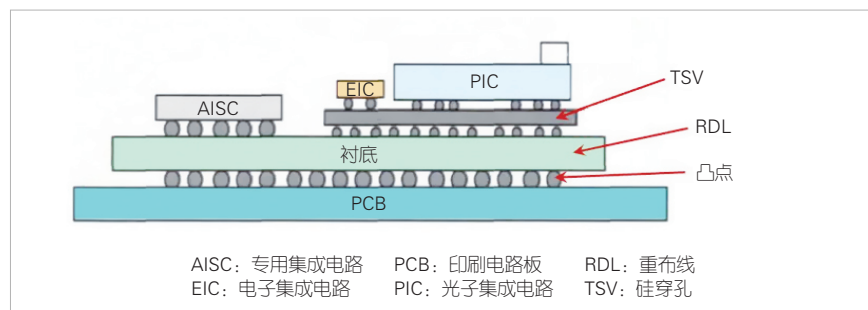
▲图5 基于带TSV的PIC转接板的共封装光学(CPO) [6]
