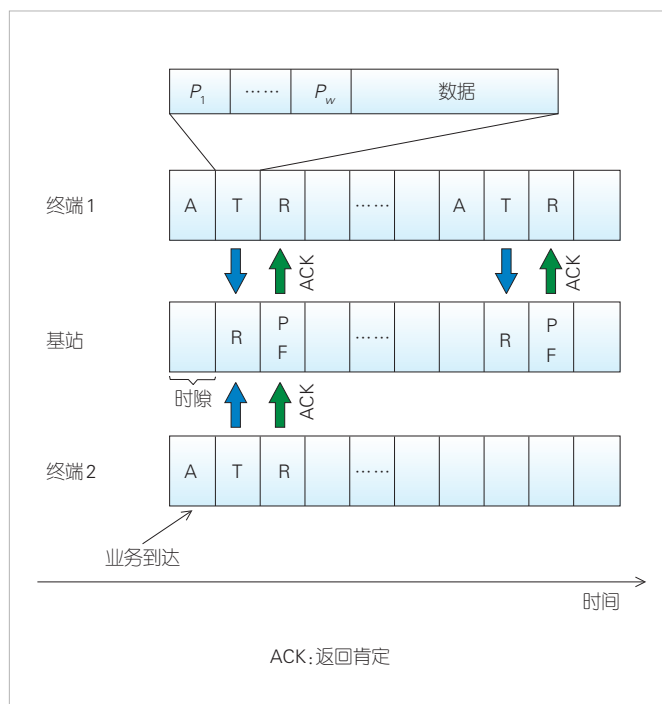
▲图1 基于竞争的无连接传输方案
