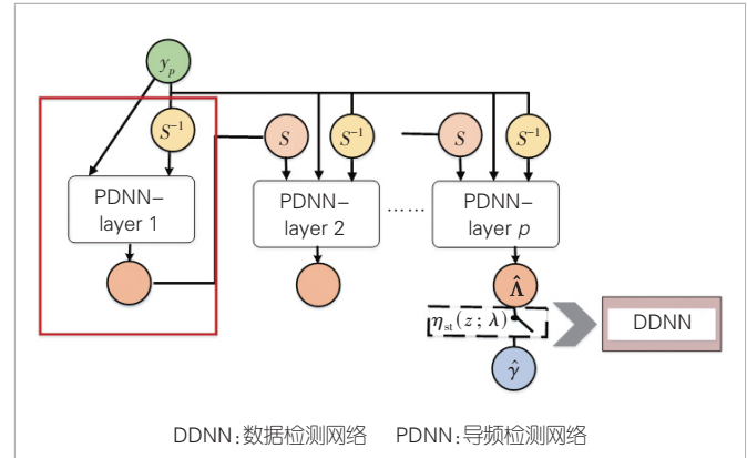
▲图7 导频检测网络示意图
