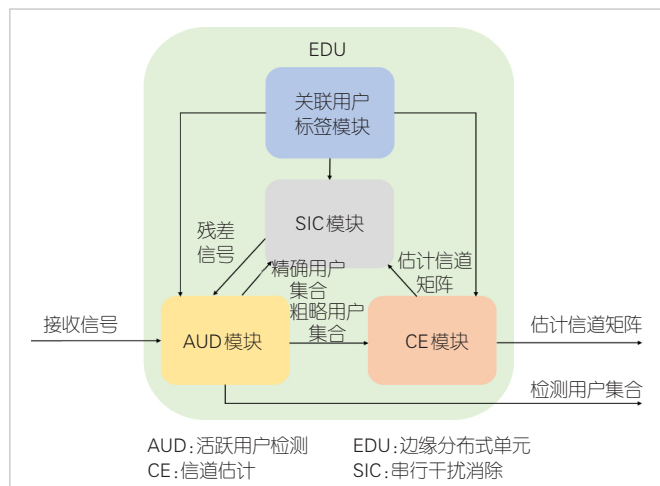
▲图3 基于SIC的联合AUD和CE处理模块示意图
