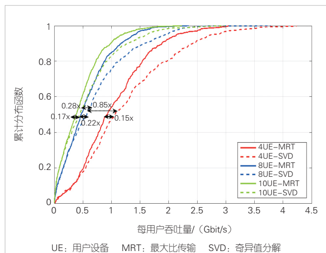
▲图 8 不同 UE 数目和不同预编码方案下 Het-LDN 的每用户吞吐量的累计分布函数(CDF)曲线
