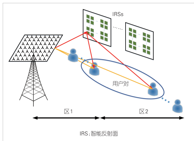
▲图3 IRS辅助的大规模多输入多输出-非正交多址用户配对
