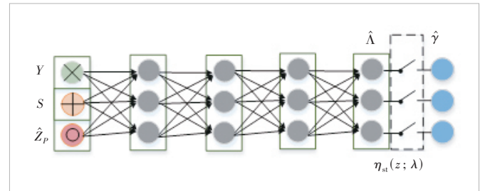
▲图8 数据检测网络示意图
