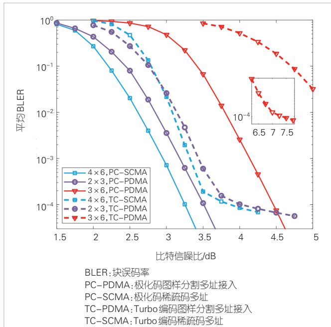
▲图4 高斯白噪声(AWGN)信道下不同配置的非正交多址接入(NOMA)方案BLER性能比较 [8]
