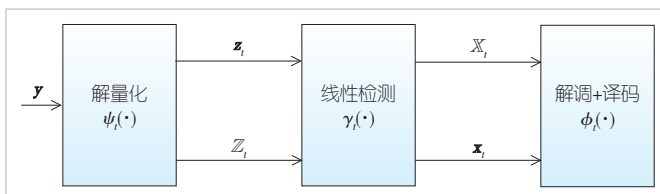
▲图8 广义AMP类接收机
