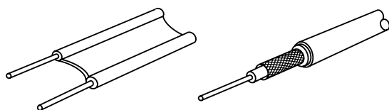
300Ωフィーダー線
