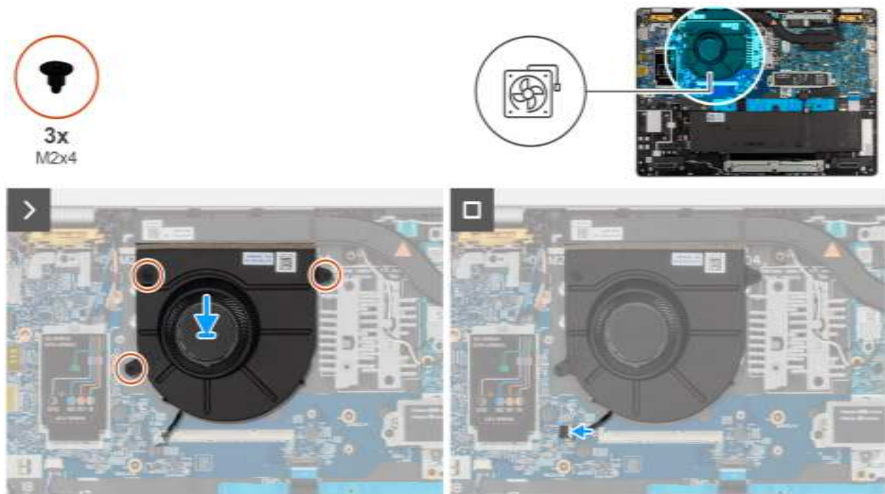
Figure 20. Installing the fan
