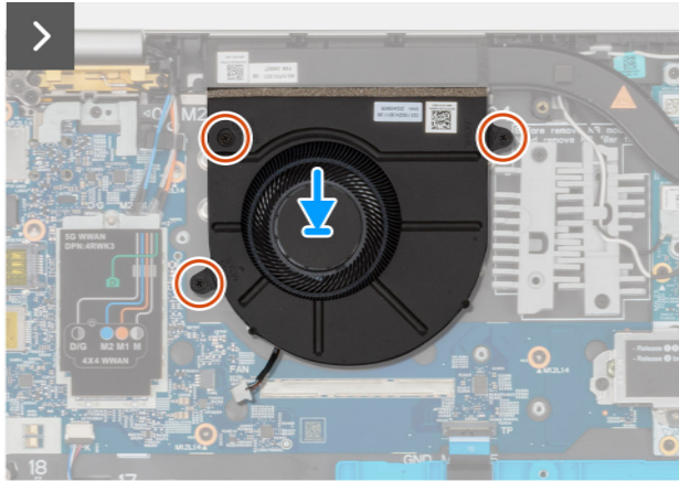
Figure 20. Installing the fan
