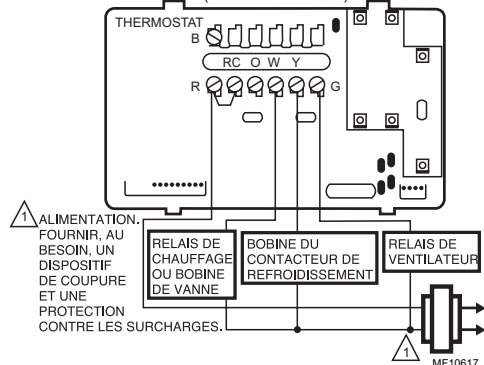
4 FILS – CHAUFFAGE/REFROIDISSEMENT (CAVALIER INTACT)
