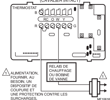
2 FILS – CHAUFFAGE SEULEMENT (CAVALIER INTACT)
