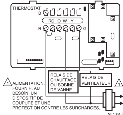
3 FILS - CHAUFFAGE SEULEMENT AVEC VENTILATEUR (CAVALIER INTACT)
