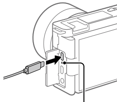
Ladekontrollleuchte
