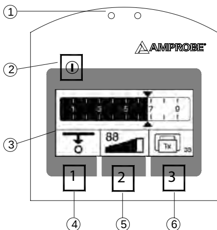
R-3500 Display
