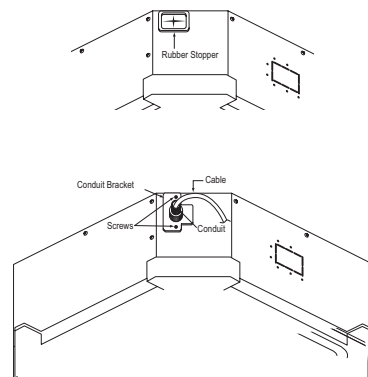
Figure 207: Using a Conduit.
