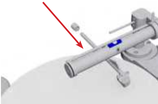
Abb. 13: Montage des Gewichtes
