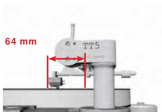
Abb. 12: Grundposition
