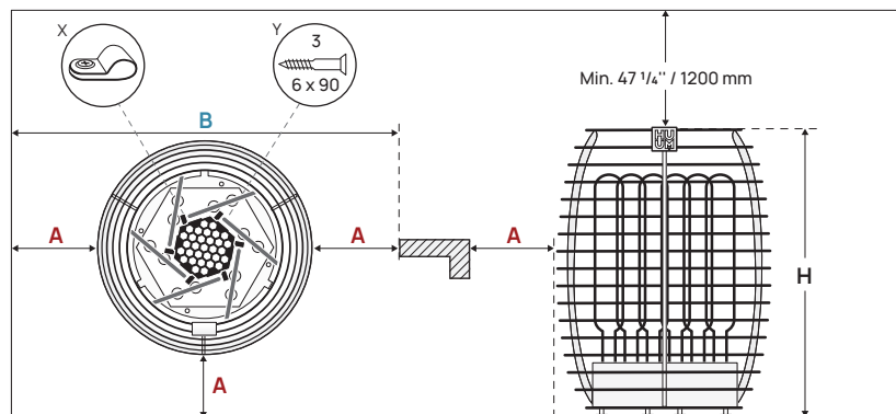
Figure 1. Positionnement du chauffe-sauna
