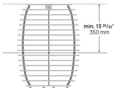
Figure 2. Installation du chauffe-sauna électrique HUUM HIVE à l'intérieur du banc de sauna
