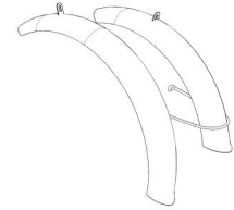
Schutzblech x 2
