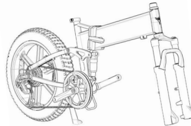
Hauptkörper
