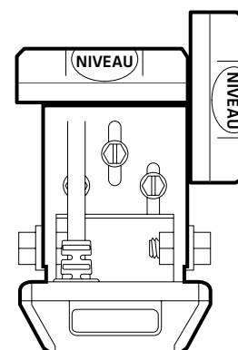
Mise à niveau du support
