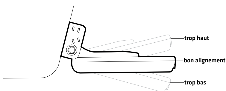
Ajustement de l'angle de fonctionnement du transducteur
