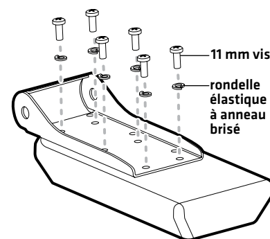
Fixation du support de transducteur
