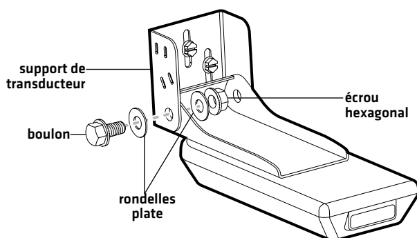
Installation du support de transducteur
