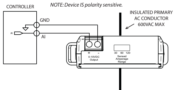
Fig. 1. Wiring CTP-5V, CTP-10V
