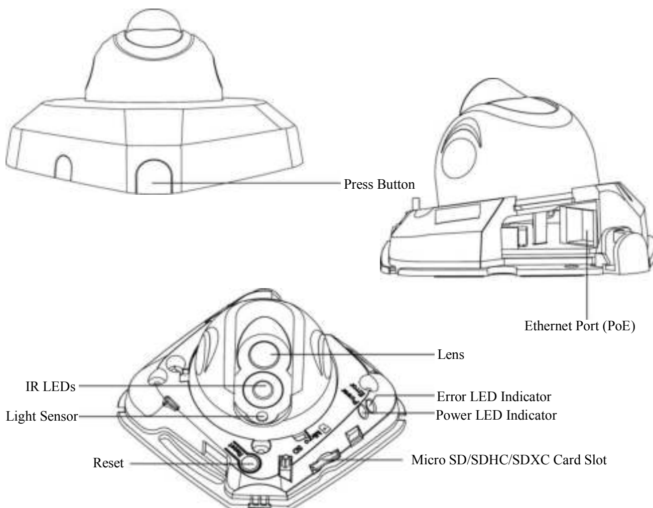
Figure 1-3-2 IR Mini Dome Network Camera
