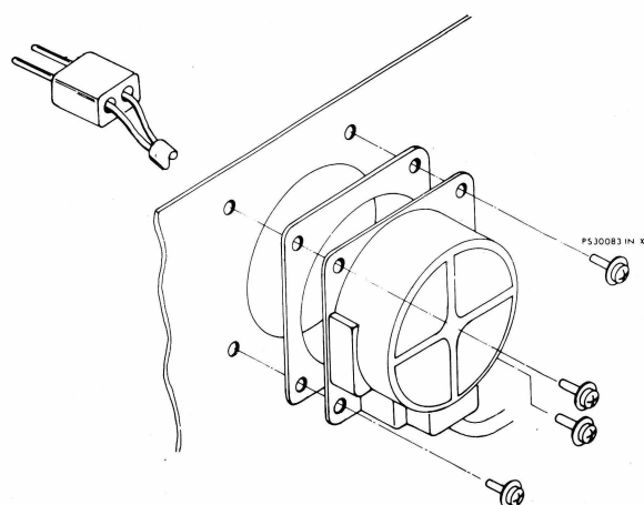
Cooling fan
