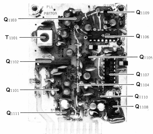
PLL unit (PB-1709A)
