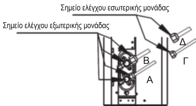
A: Βαλβίδα απομόνωσης χαμηλής πίεσης B: Βαλβίδα απομόνωσης υψηλής πίεσης Γ & Δ: Ρακόρ εσωτερικής μονάδας
